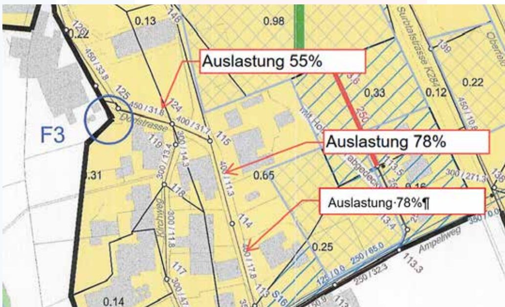
Abbildung 2: Auslastung Kanalisation (2026) GEP (2008)
